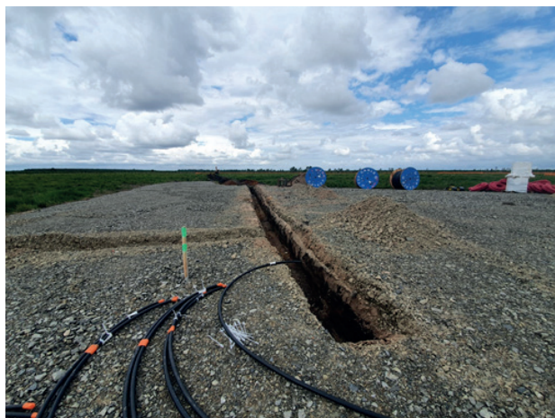
Installation du réseau de câbles interne au parc
